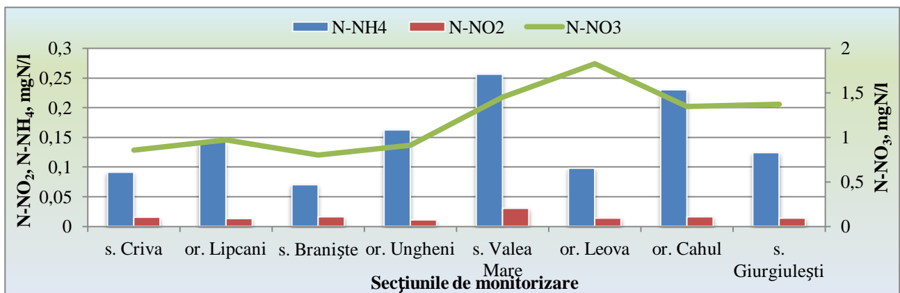
Figura 2. Percentila 90 pentru elementele biogene din grupa azotului pentru anul 2015 în secțiunile de monitoring ale r. Prut
